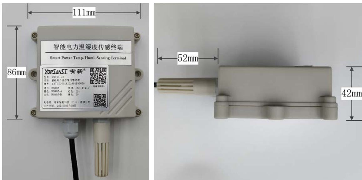
图 2-1 外观示意图
